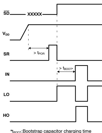
Figure 35. POR Sequence
